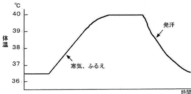
図1 感染症にかかったときの体温変化と身体反応の時間経過
