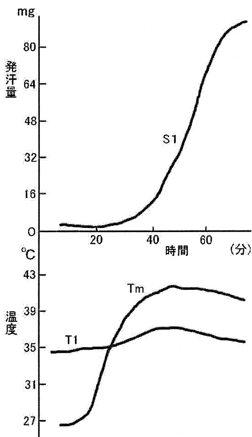
図2 室温（Tm）を変化させたときの胸部の発汗量（S1）と皮膚温（T1）の変化
