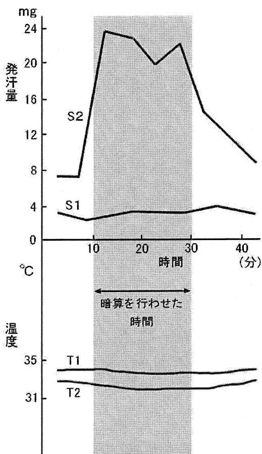
図3 暗算を行わせたときの胸部の発汗量（S1）と皮膚温（T1）、手のひらの発汗量（S2）と皮膚温（T2）
